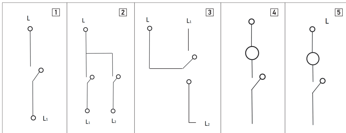
Рисунок 1. Электрические схемы выключателей серии DITA
