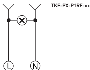
Рисунок 1. Электрические схемы подсветки серии PIXEL (ТОКОВ™).
