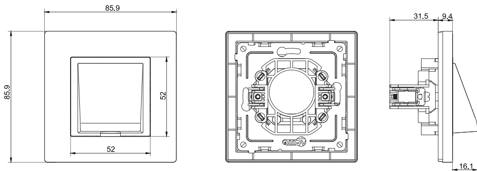
Рисунок 2. Габаритные размеры схемы вывода кабеля серии PIXEL (ТОКОВ™).
