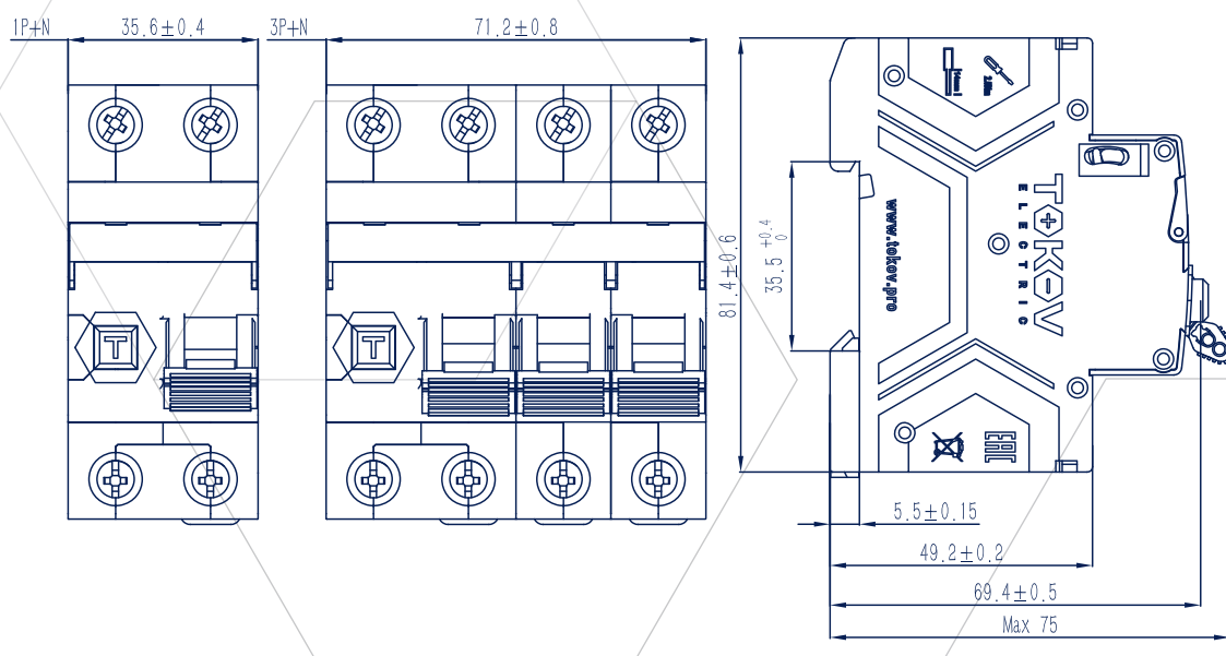
Габаритные размеры
